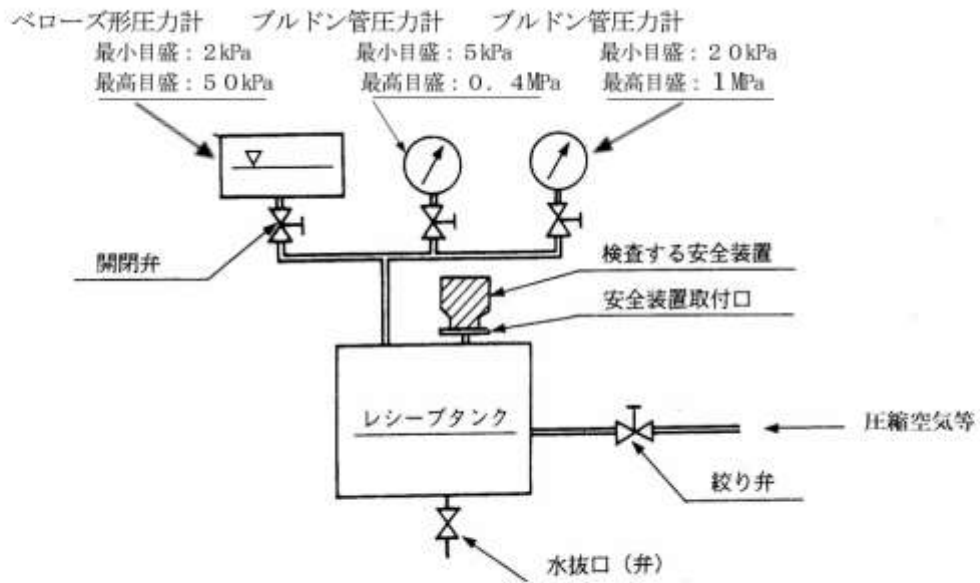
例1 最高試験圧力1MPaの試験装置
